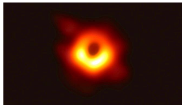
ブラックホール画像(国立天文台 HP より)
