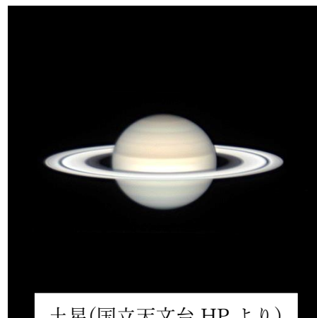
土星(国立天文台 HP より)
